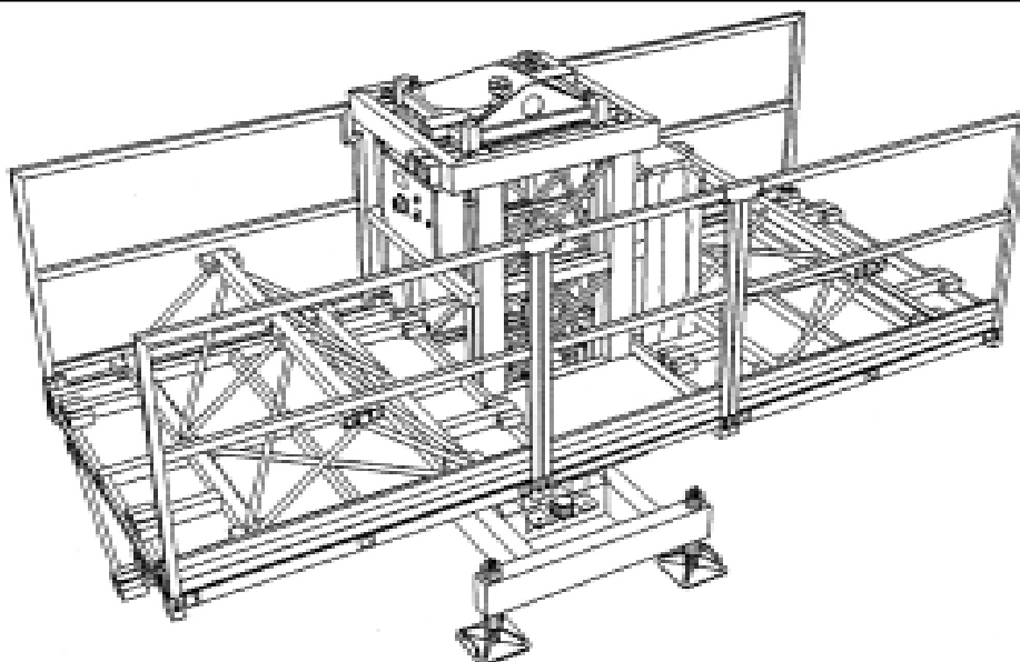
Рисунок 7.4. 2 боковые помосты.
