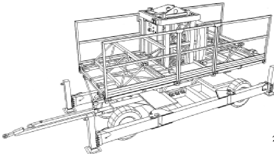
Рисунок 7.2. 2 боковых помостов.
