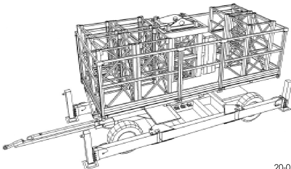
Рисунок 7.3. 6 секций мачты.
