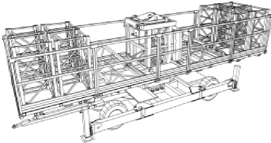
Рисунок 7.1. 8 секций мачты и 2 боковых помостов.
